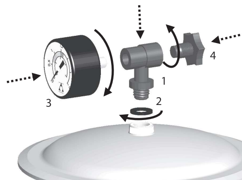
Montage du manomètre (avec le bouchon de dégazage d'eau)
