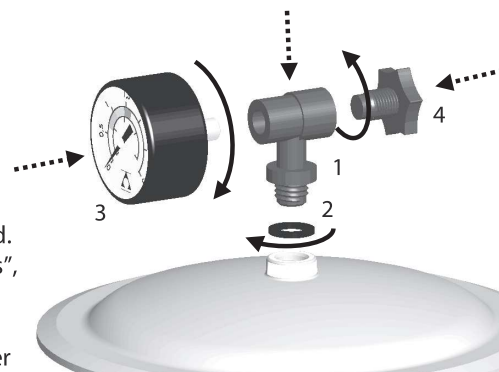
Montage des Manometers (mit Entlüftungsventil)
